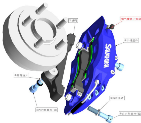
左后轮卡钳安装图
